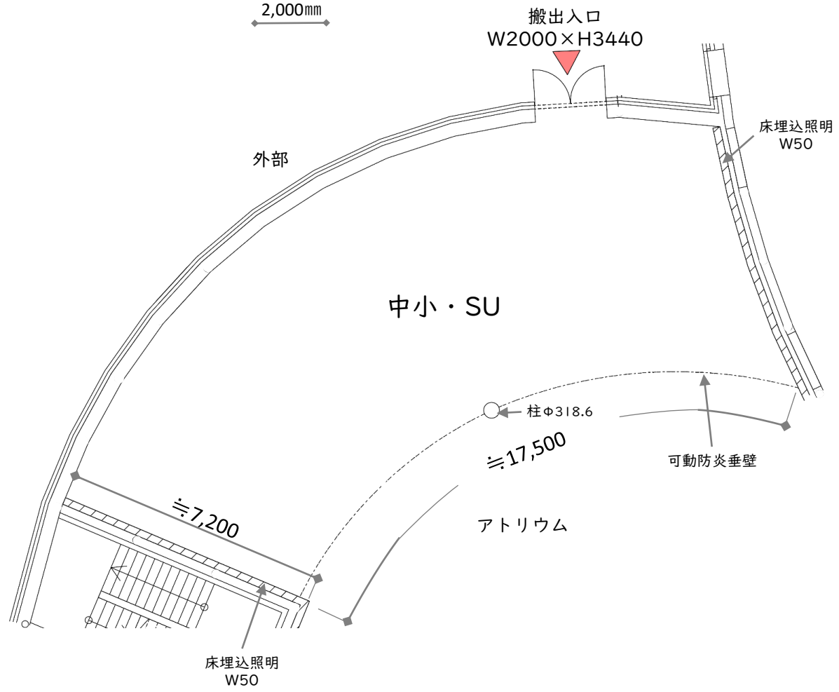
平面図 A4: 1/150
