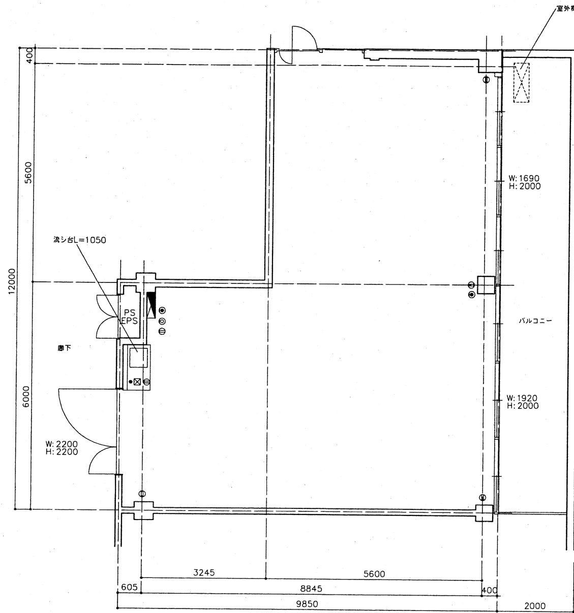
3階 95.1m 2 のユニット平面図 (貸室番号 301)
