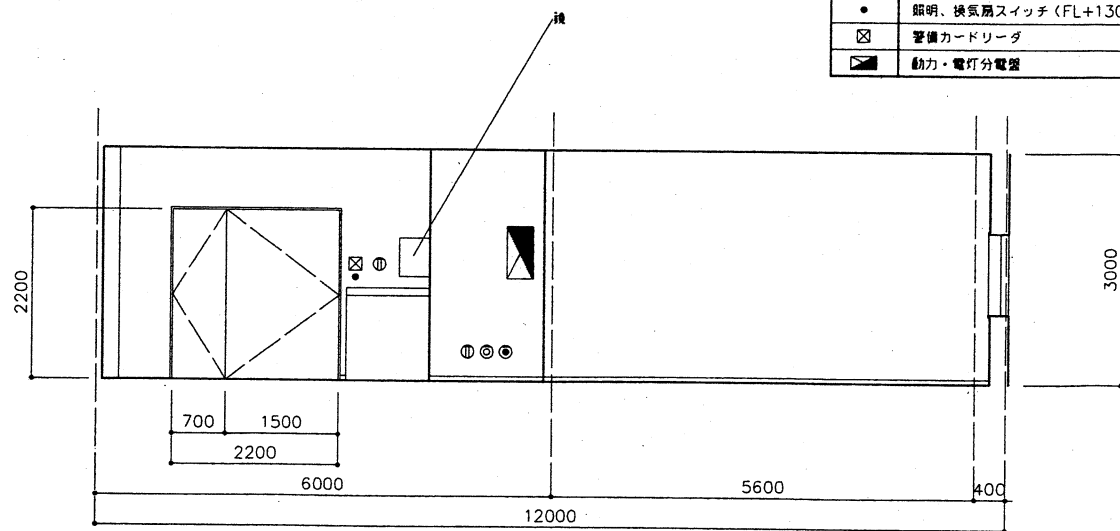
3階 95.1m 2 のユニット平面図 (貸室番号 301)
