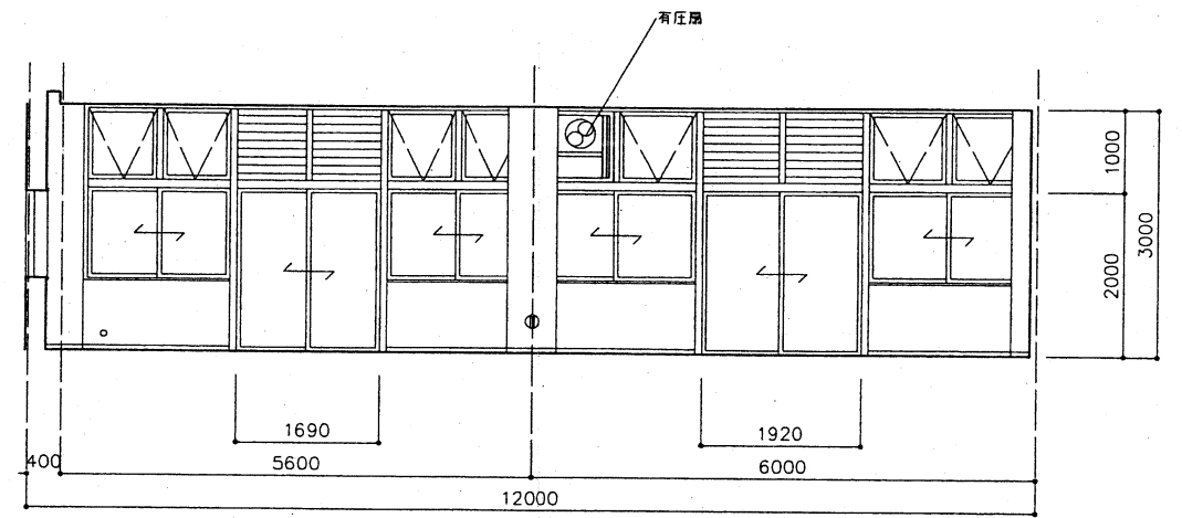
B 展開図
