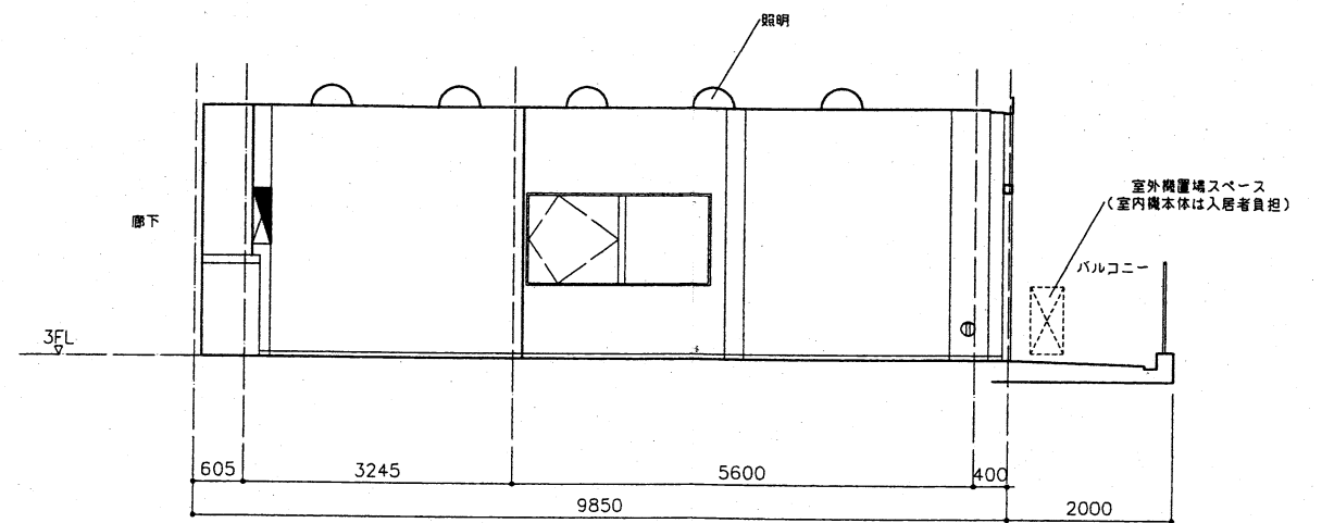
A 展開図
