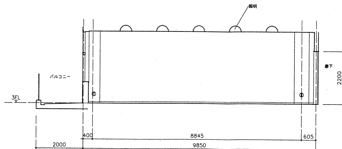
C 展開図
