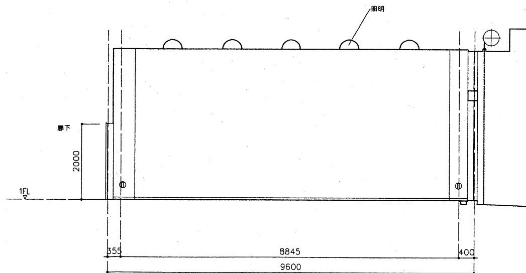
C 展開図
