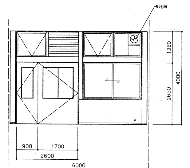
D 展開図
