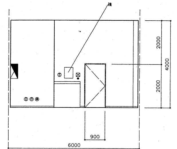
B 展開図
